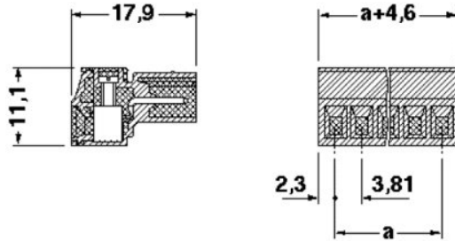
Maßzeichnung
