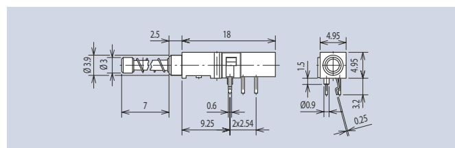
Ausführung 1446 ... · Version 1446 ...
