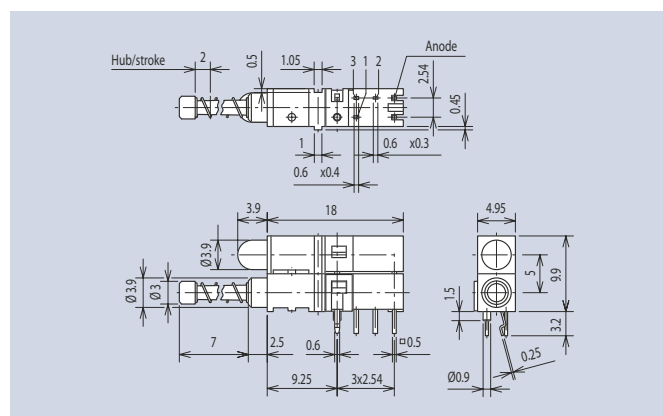
Ausführung 1445 ... · Version 1445 ...
