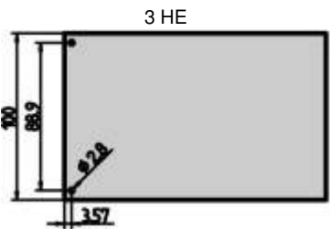
Bohrungsmaße auf der Leiterkarte
