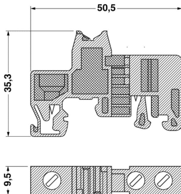
Maßzeichnung
