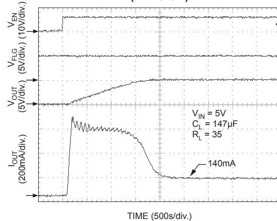
Turn-On (MIC2026-1)
